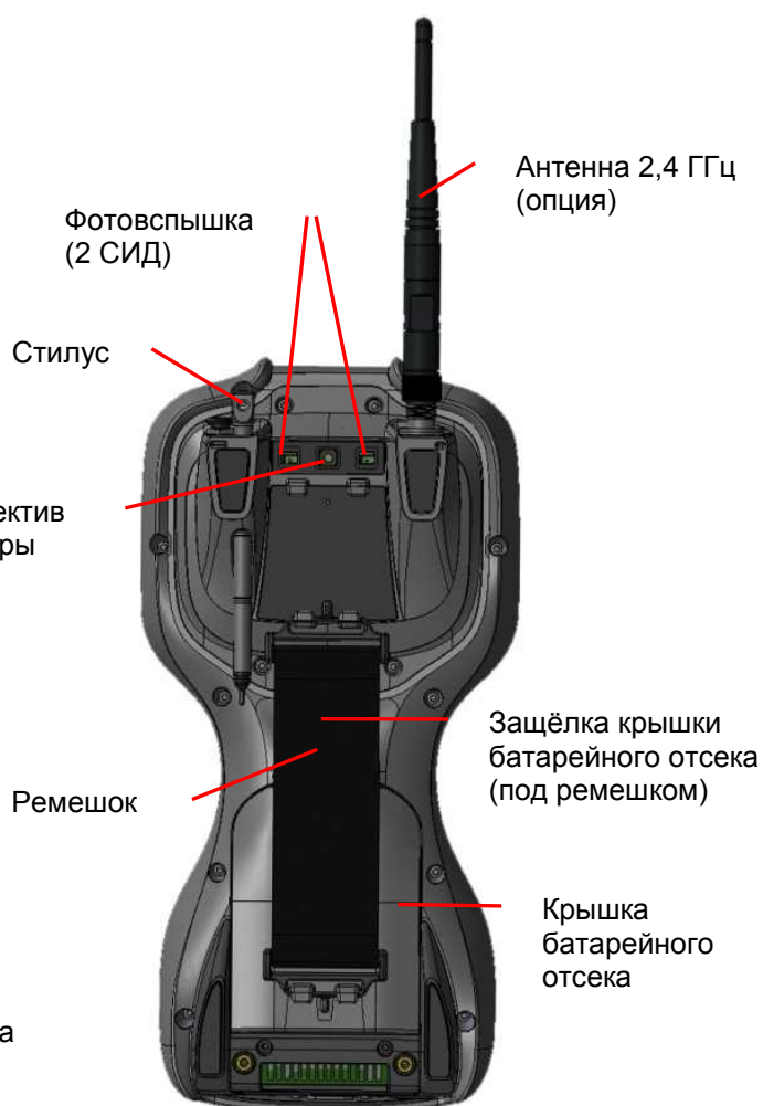
Вид сзади
