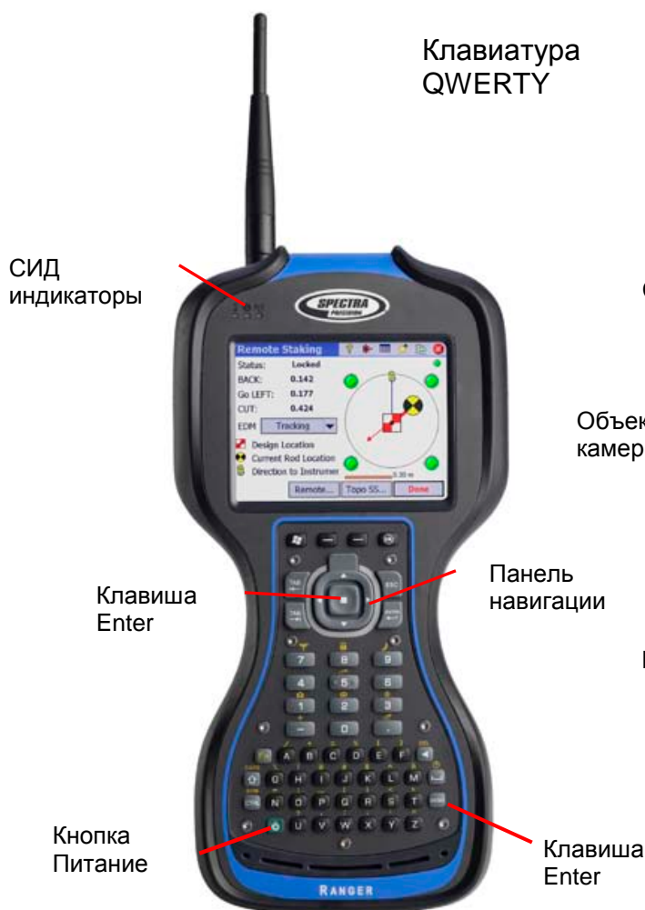
Вид спереди
